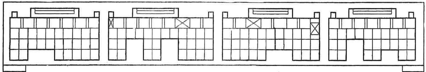
4カプラ 135ピン Cタイプ
