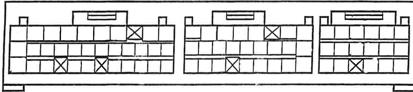
3カプラ Aタイプ
